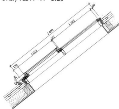
svislý řez A - A 1:20
