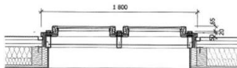
vodorovný řez B - B 1:20
