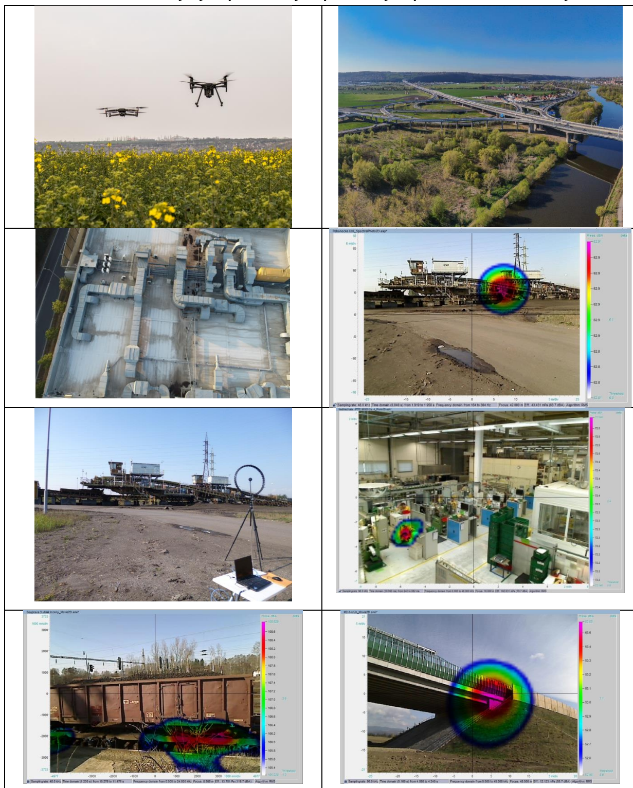
Obr. 2: Příklady výstupů leteckých prací a výstupů z akustické kamery
